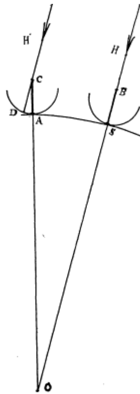
Figure 3 : Schéma représentant la méthode d'Eratosthène telle que décrite par Cléomède. L'arc AD est égal à 1/50^e du cercle de centre C et de rayon [AC]. Comme les angles C et O sont égaux, l'arc AS délimite 1/50^e du cercle terrestre.
